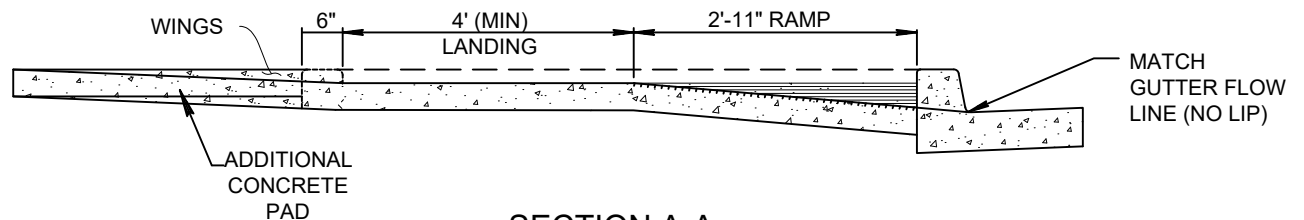
SECTION A-A
